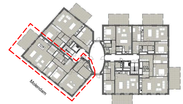
Grondplan
